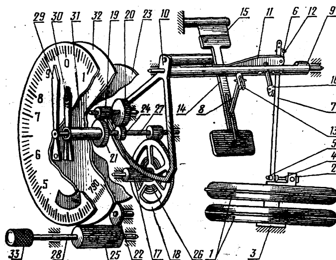
Кинематическая схема высотомера ВД
